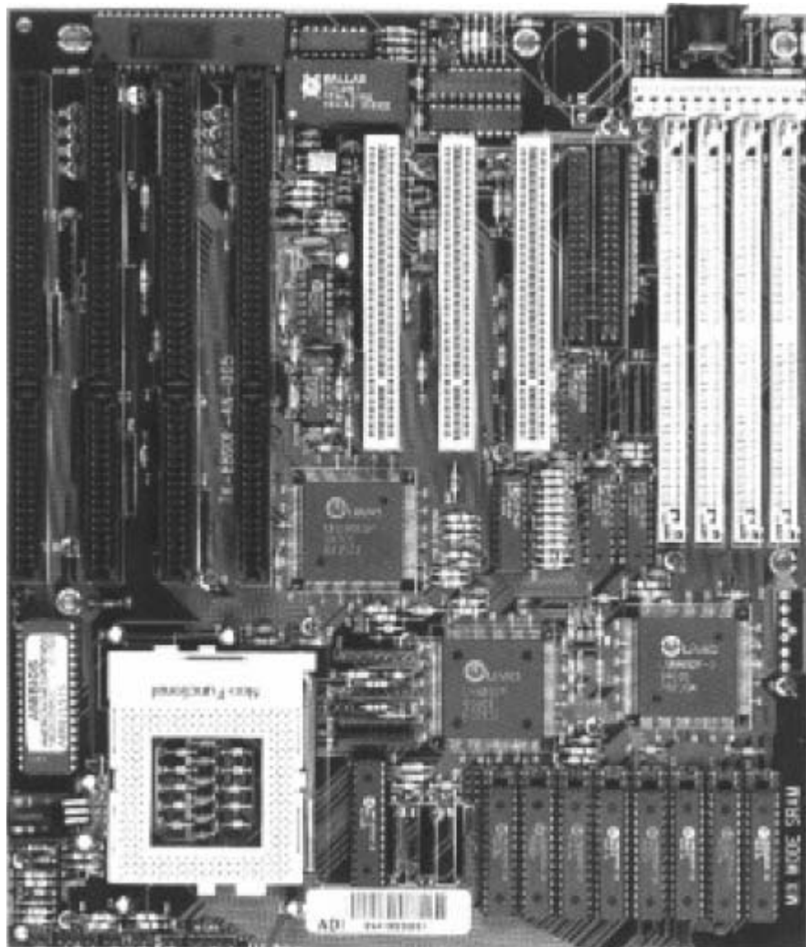
Figura 14 - Placa de CPU
